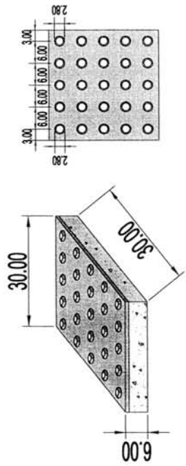
ТИП "А" - плоча узорчења
