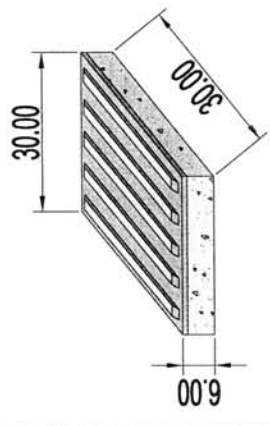
ТИП "Б" - плоча водилџа за слепа и слабовиде
